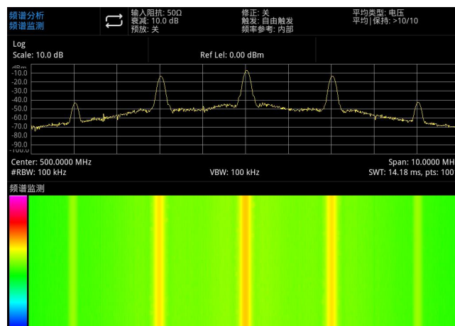
图 5-6：频谱监测
