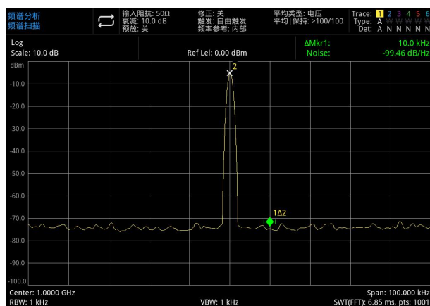
图 3-20: 相位噪声
